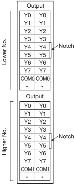
FX5-C32EYT/D
