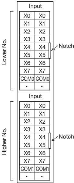
FX5-C32EX/DS
