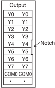
FX5-C16EYT/D
