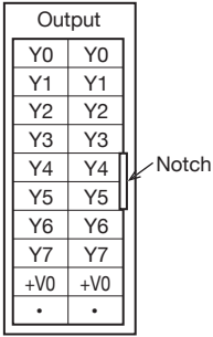
FX5-C16EYT/DSS
