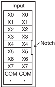
FX5-C16EX/D
