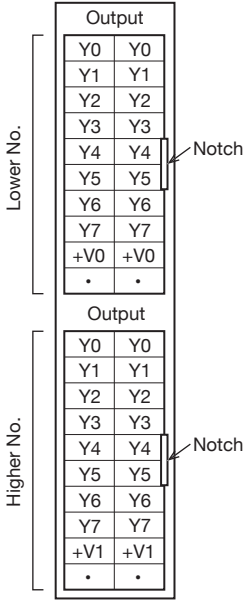
FX5-C32EYT/DSS
