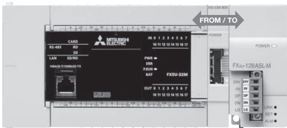
FX3U-128ASL-M
