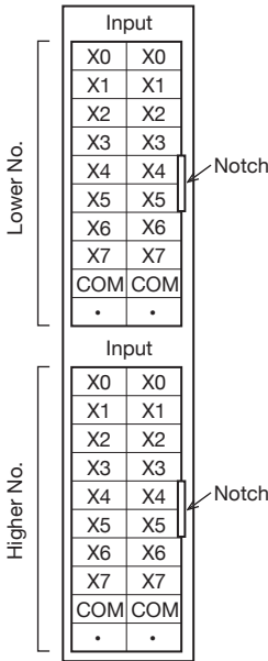
FX5-C32EX/D
