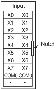
FX5-C16EX/DS
